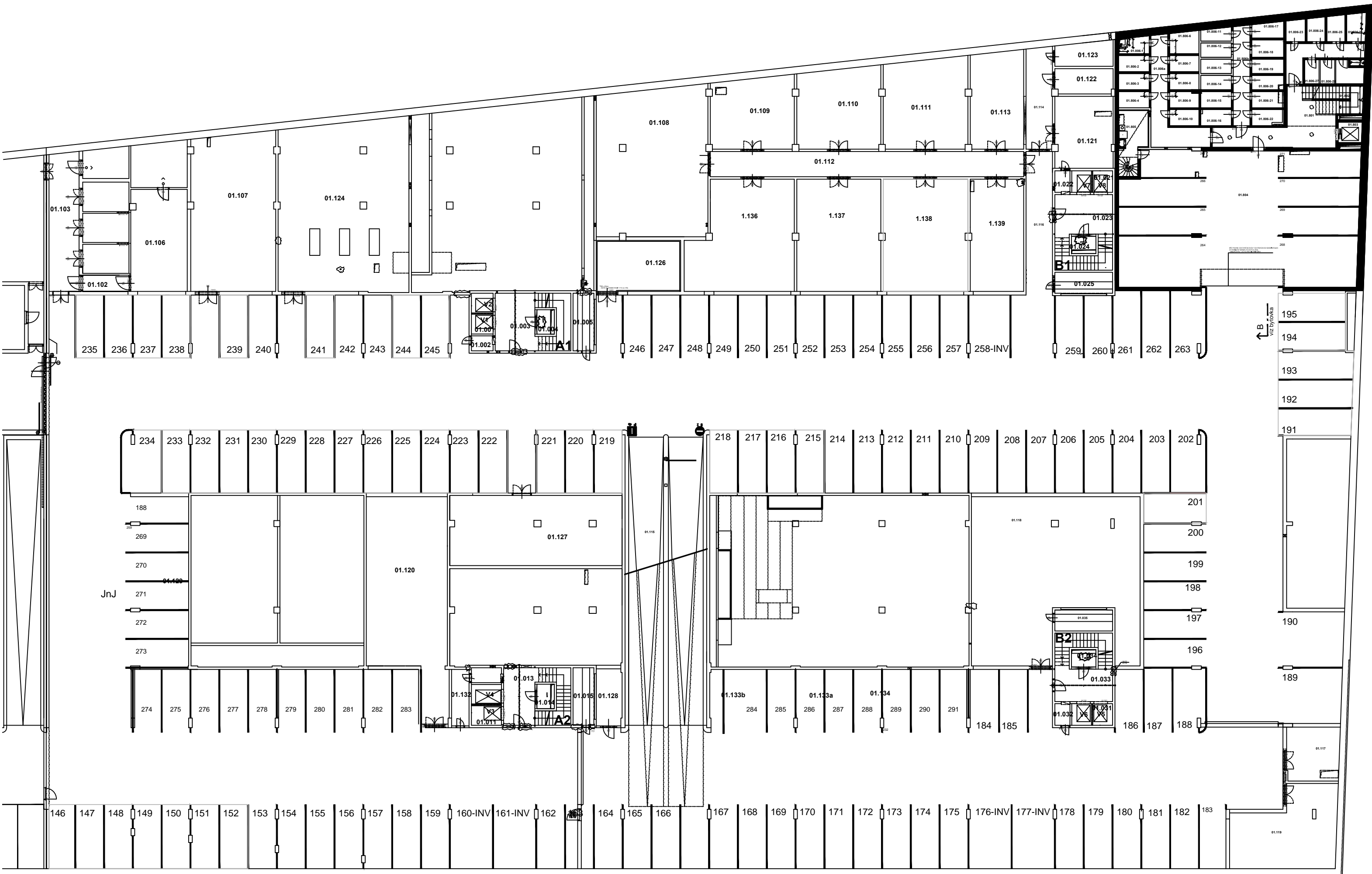
PŪDORYS 1. SUTERĒN M 1:275
